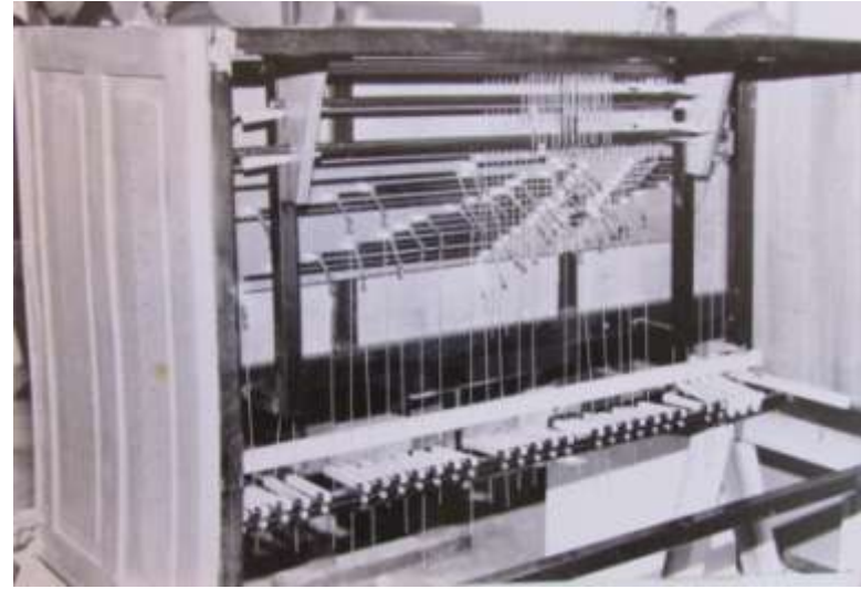
Mécanisme d'un orgue de salon en construction
